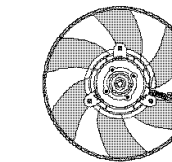
822 03 02 Lüfter kpl. 300 mm 1.4i; 1.6i; 1.7 SDi; 1.9 SDi
